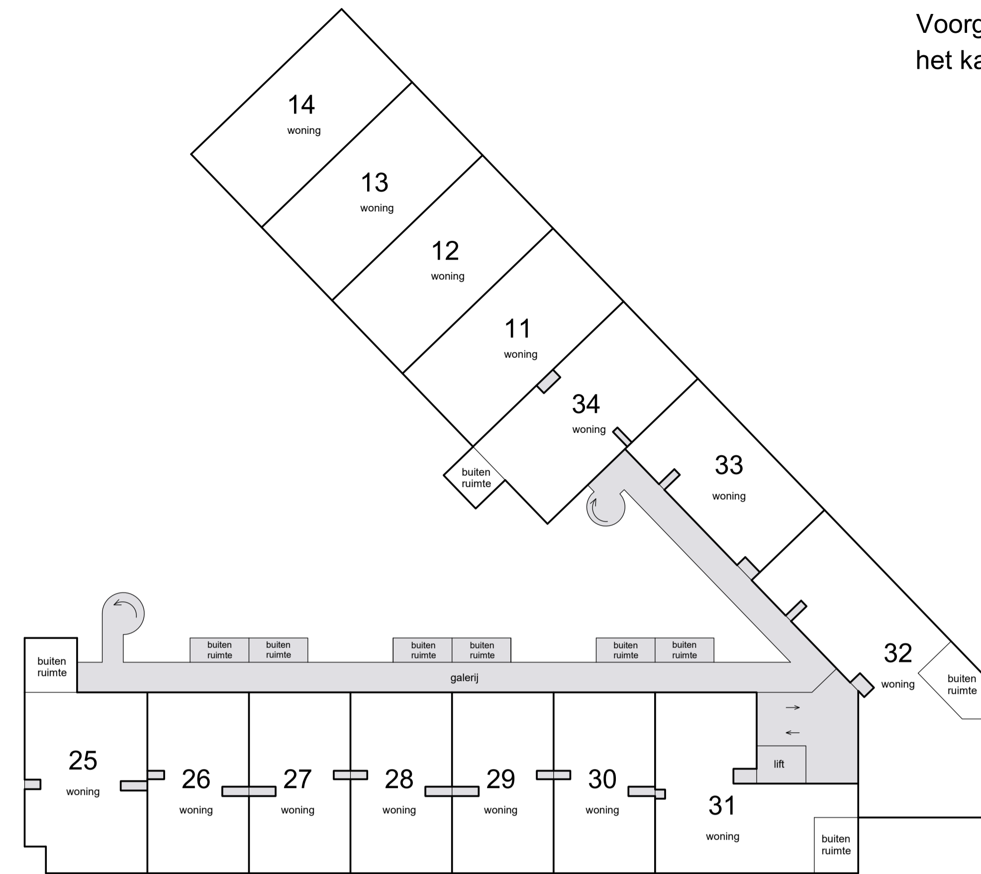
2e etage
