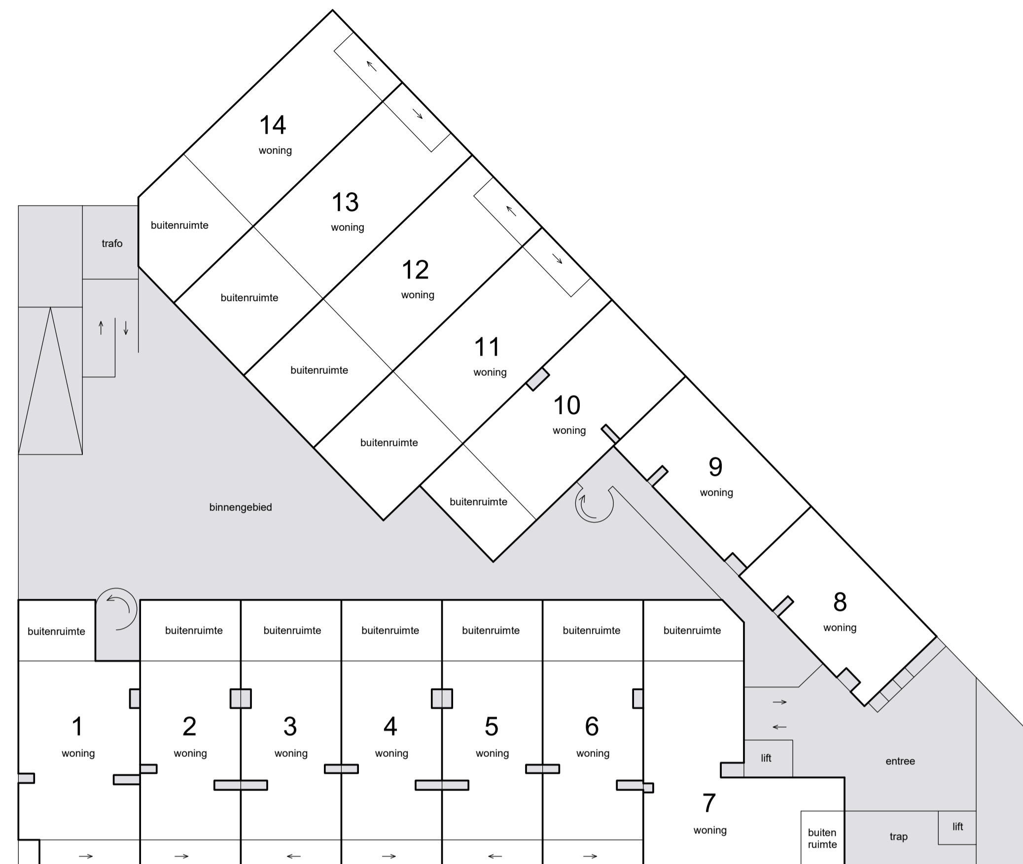
begane grond
